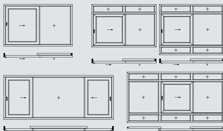
Sheme otvaranja kliznih stijena PremSlide 76
